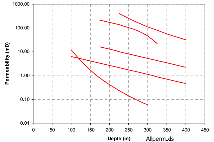
Fig. 2 – Example Actual Permeability Gradients
