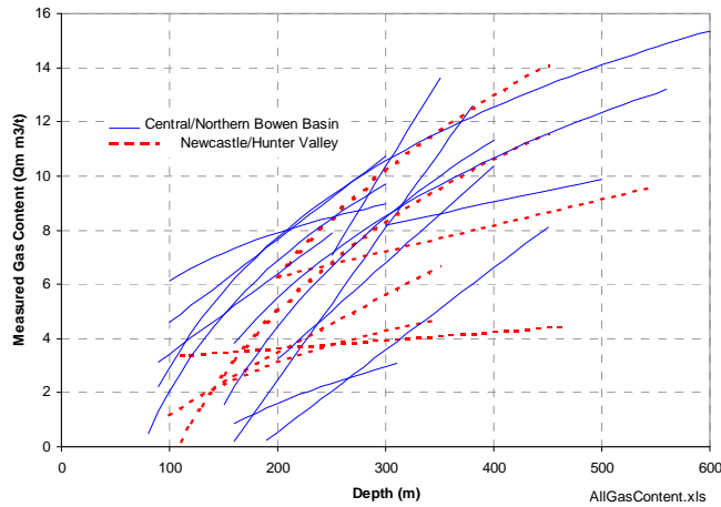
Fig. 1 – Example Actual Gas Content Gradients
